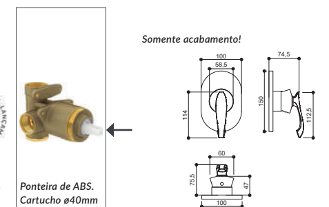
Ref. RB88090 Acabamento rose gold. Não acompanha a base Deca Ref. 4493. Base com cartucho de 40mm.
