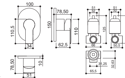
Ref. KR82670 Misturador monocomando para chuveiro. Base com cartucho de 40mm. Entrada de 3/4". Acabamento rose gold [40837]. Acompanha base.
