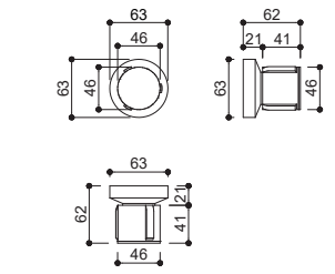
Ref. KR8192F Para base Fabrimar. Acabamento rose gold [37396].
